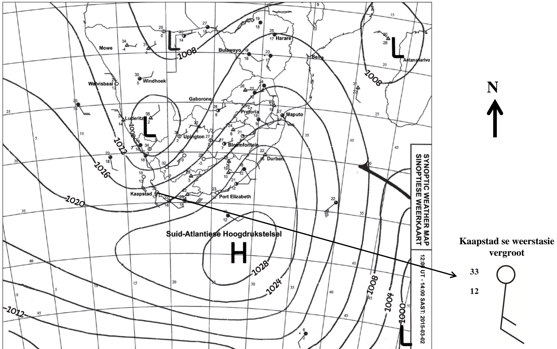
Figuur 2: Sinoptiese weerkaart, 2 Maart 2015
